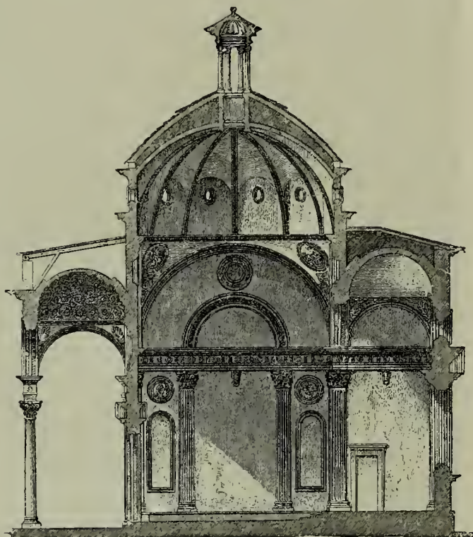
Abb. 88 und 89. Capp. Pazzi zu Florenz.
